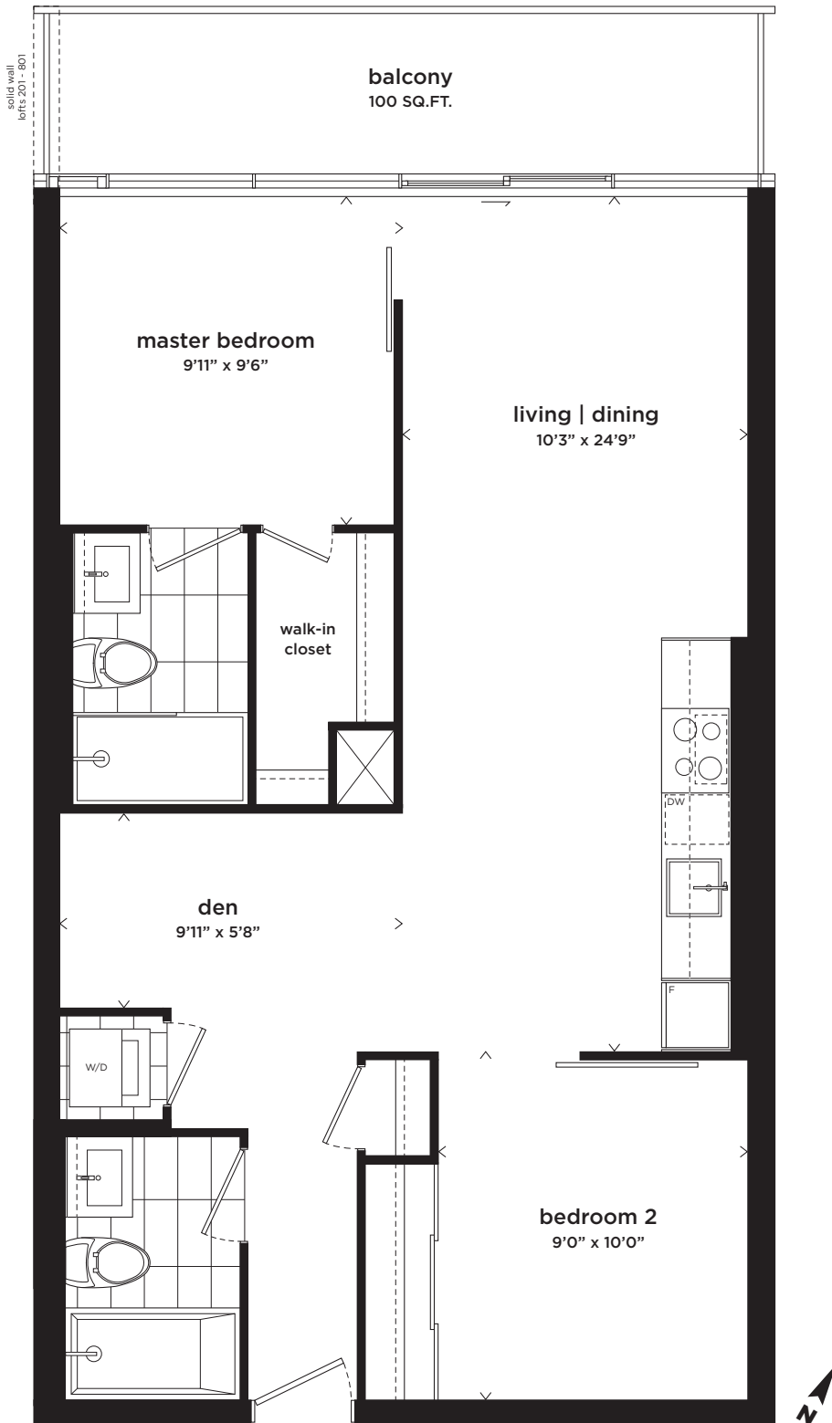
LOFTS 202 - 802 SHOWN
